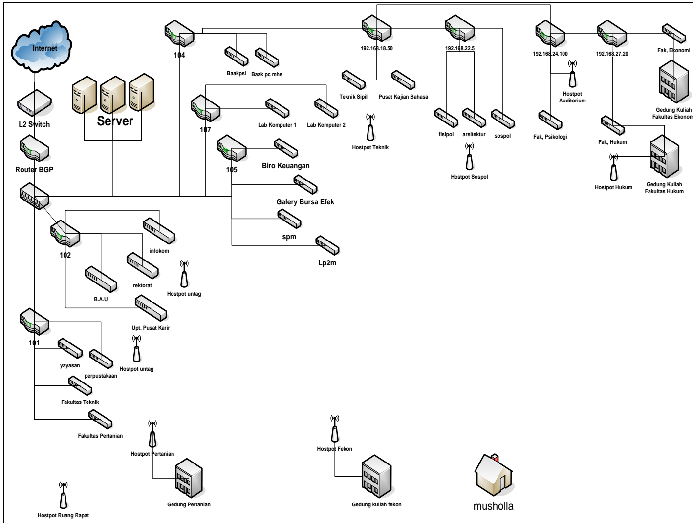
Gambar 3.1. Topologi Jaringan UNTAG 1945 Samarinda Tahun 2018
