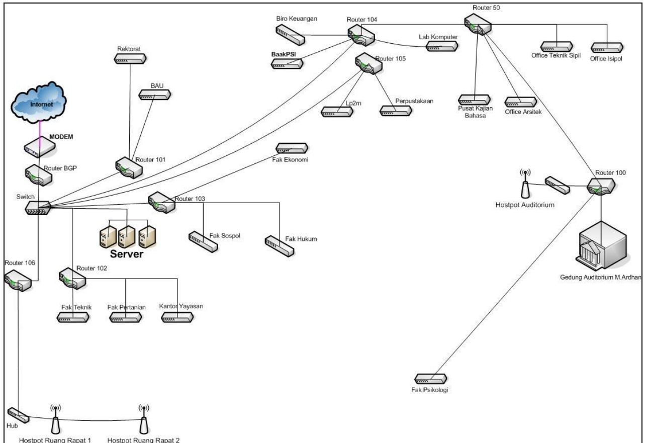
Gambar 3.2. Rancangan Topologi Jaringan Untag 1945 Samarinda
